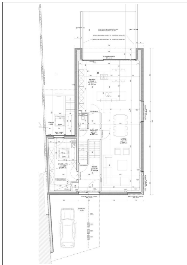
Gelijkvloers
