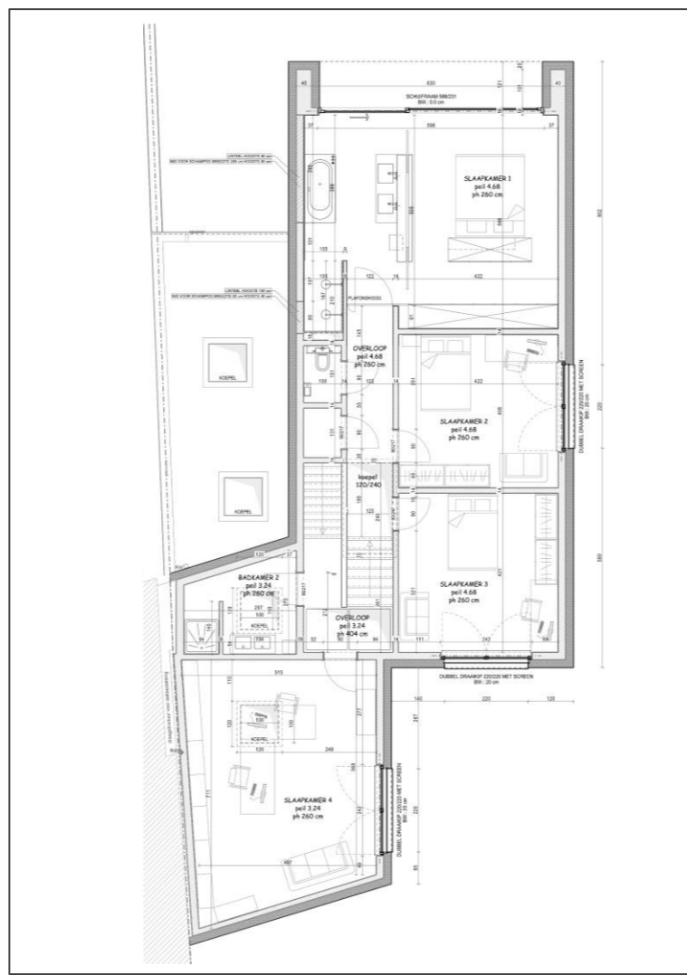
Eerste verdieping
