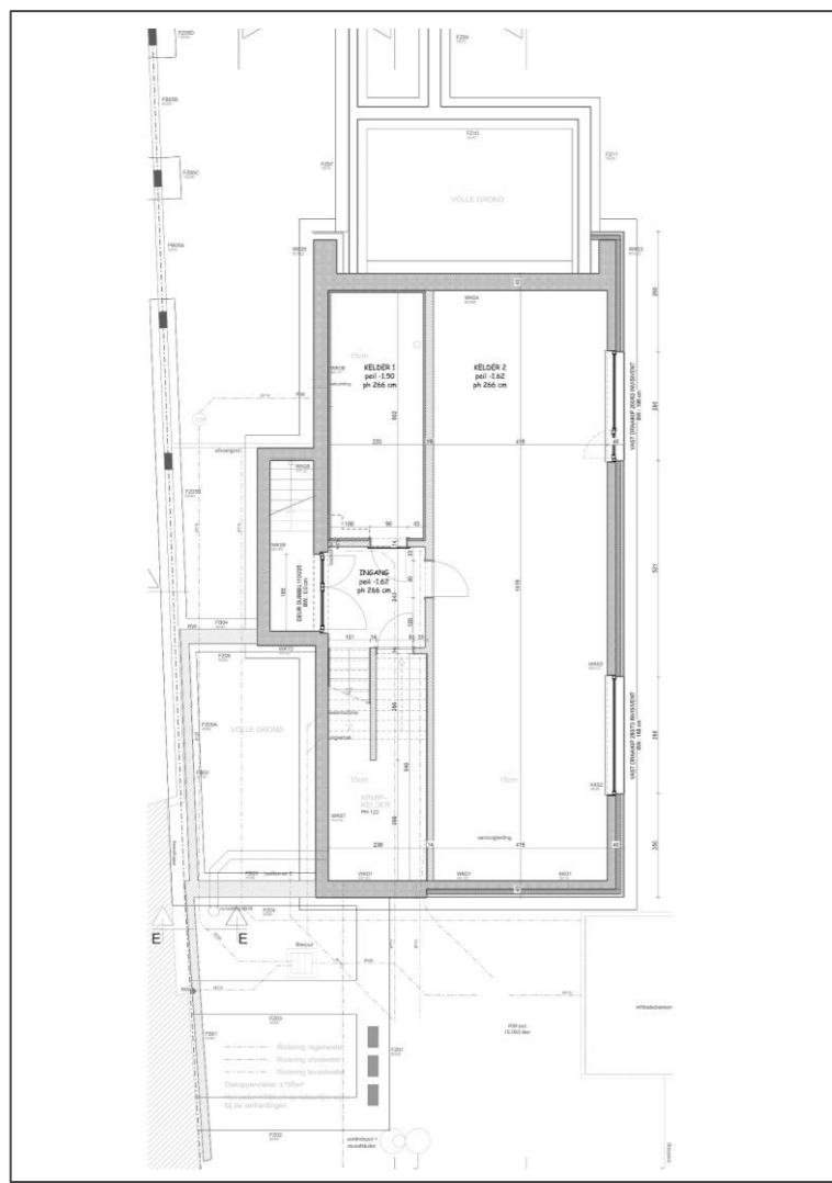
Kelderverdieping
