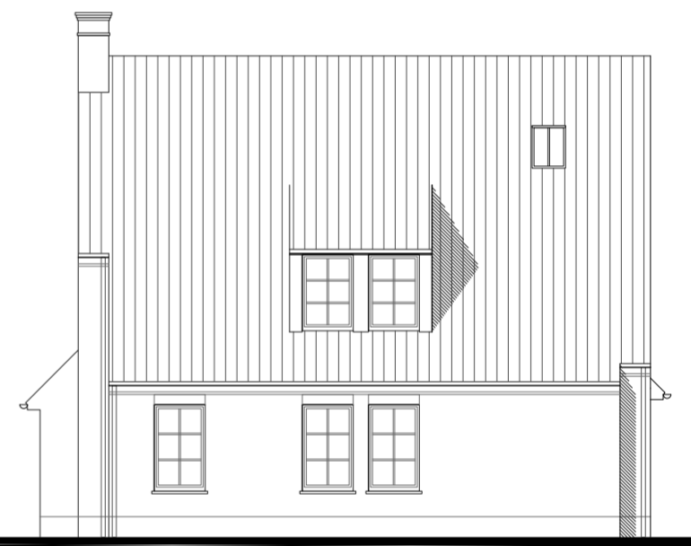
zijgevel rechts LOT 2
