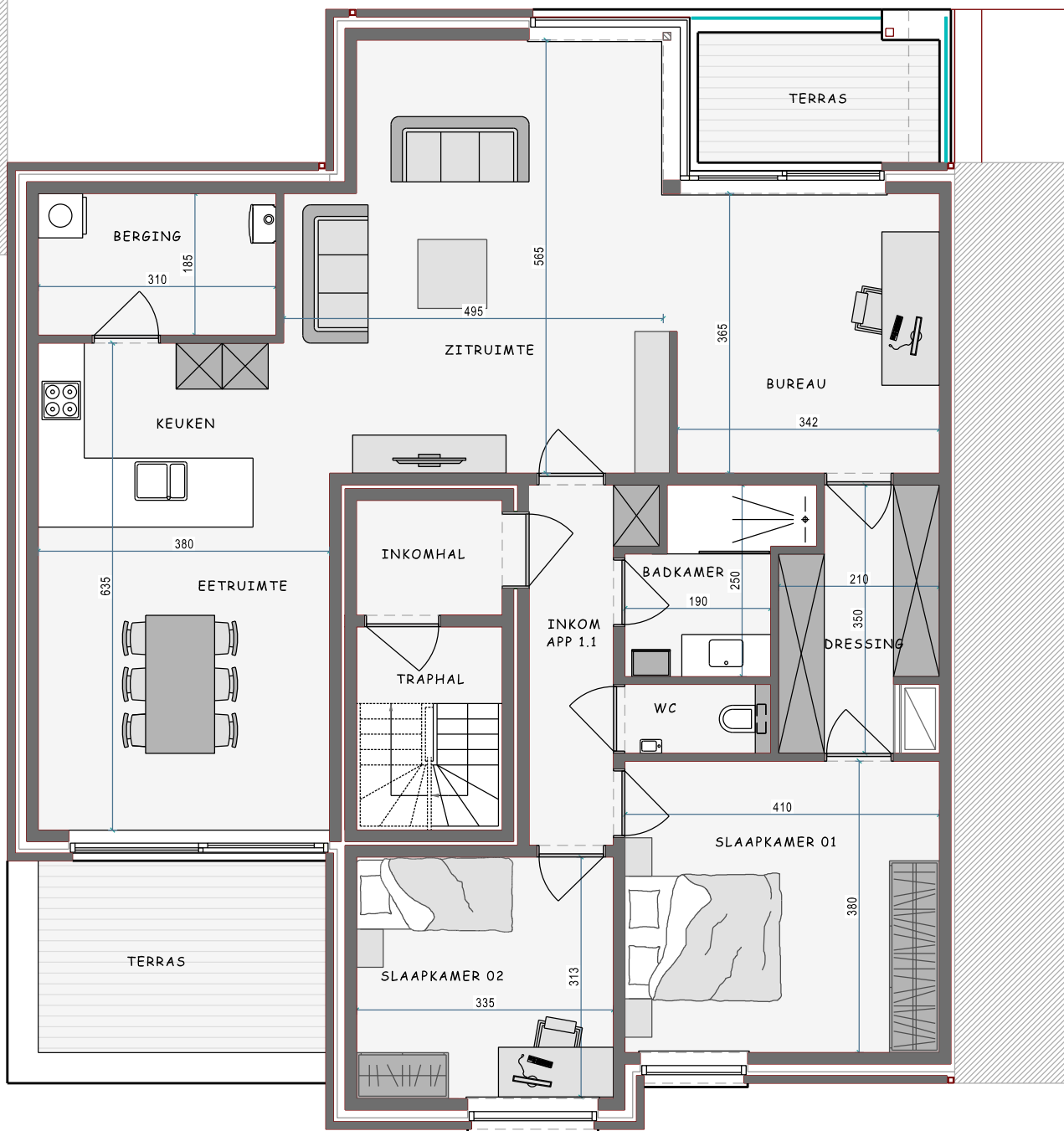
PLAN VERDIEPING 01 HERMITAGESTRAAT
